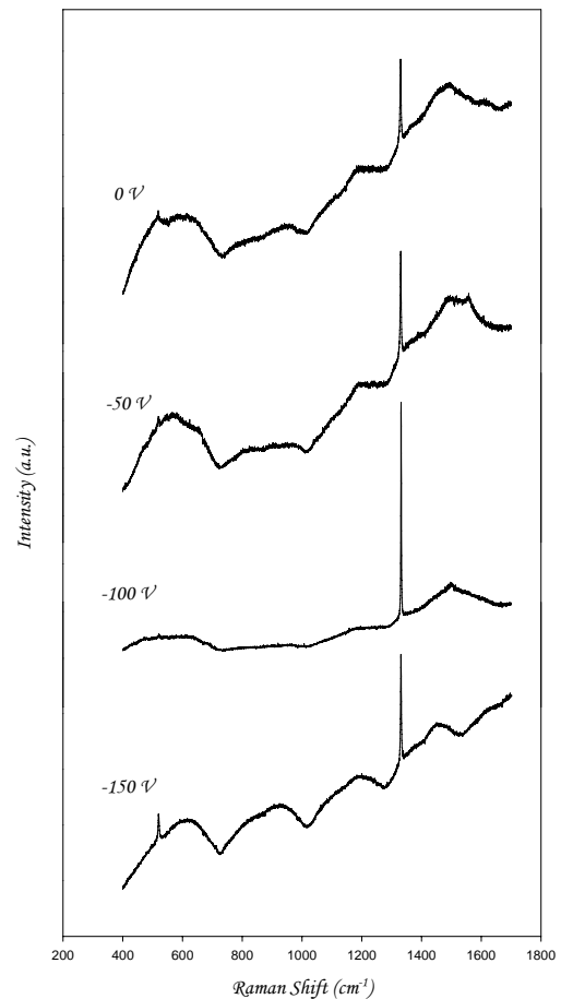
圖 7. 改變 BEN 的偏壓大小所得到多晶鑽石之拉曼光譜圖
