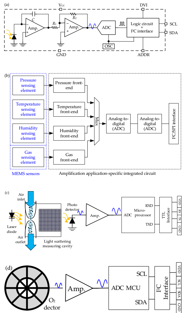
圖 2.2 多元、異質感測器方塊圖
