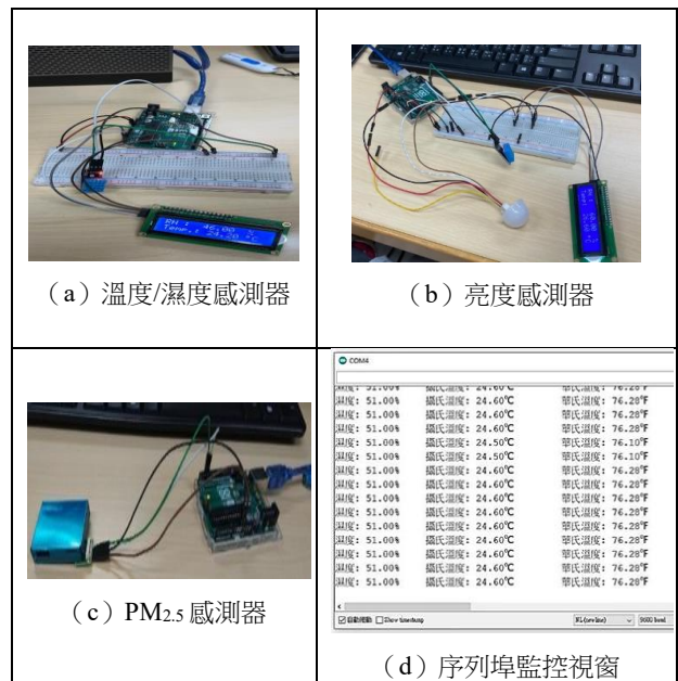
圖 3.2 連接 Arduino Uno 平台端實作照片
