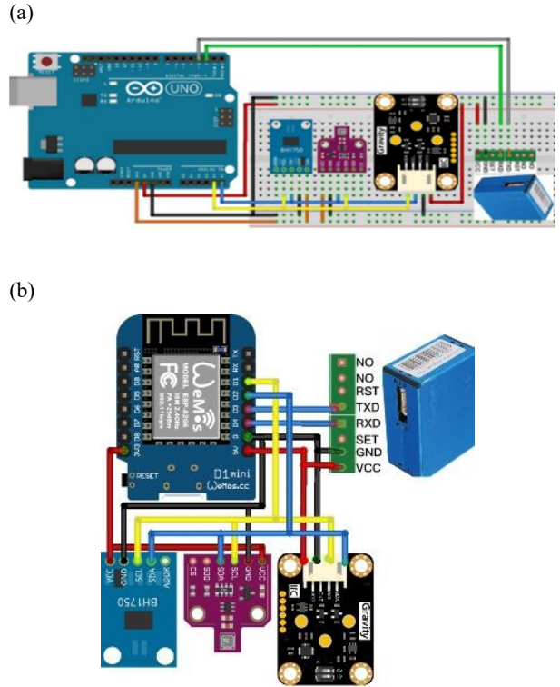
圖 3.1 多元、異質感測器元件接線圖
