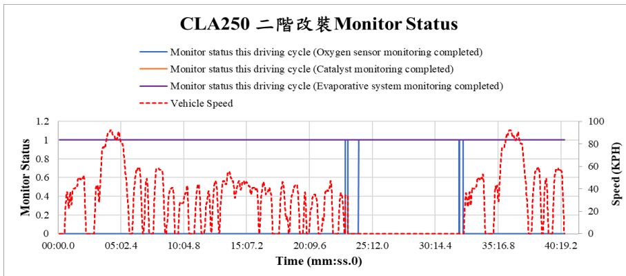
圖 14. CLA250 二階改裝 ECU 軟體之各監控系統就緒情形
