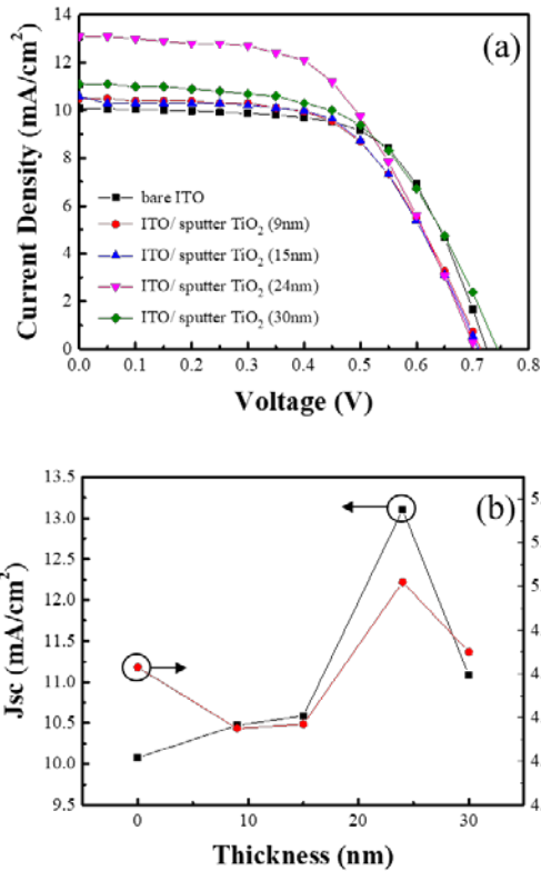
圖 7. (a) 調變 TiO 2 緻密層厚度之 DSSC 元件 J-V 曲線圖、 (b) 調變 TiO 2 緻密層厚度之短路電流密度與光電轉換效率
