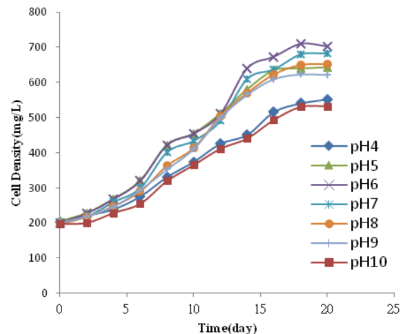
圖 7. 不同 pH 下，小球藻之生長曲線
