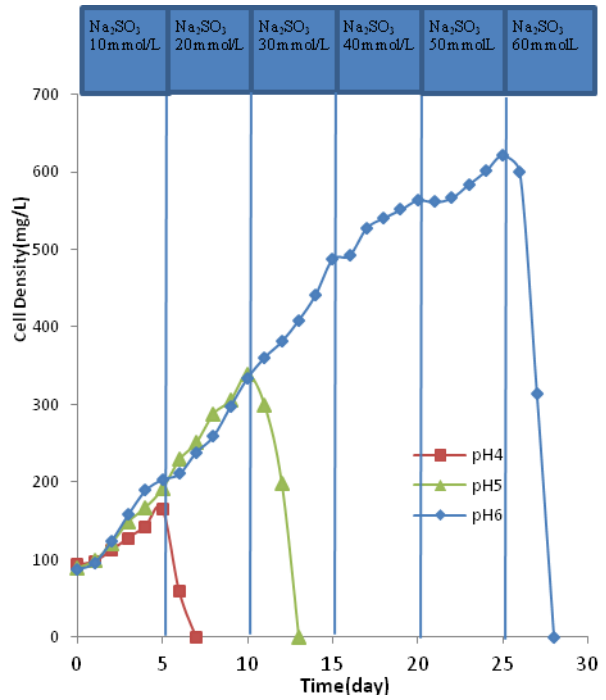
圖 10. 小球藻對 Na 2 SO 3 忍耐力
