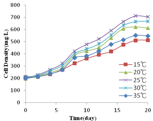
圖 8. 不同溫度下，小球藻之生長曲線
