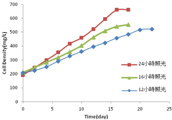
圖 9. 不同照光時間下，小球藻的生長曲線之影響
