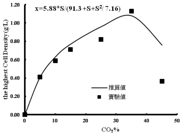
圖 5. 不同濃度 CO 2 培養下，小球藻之最高生長濃度
