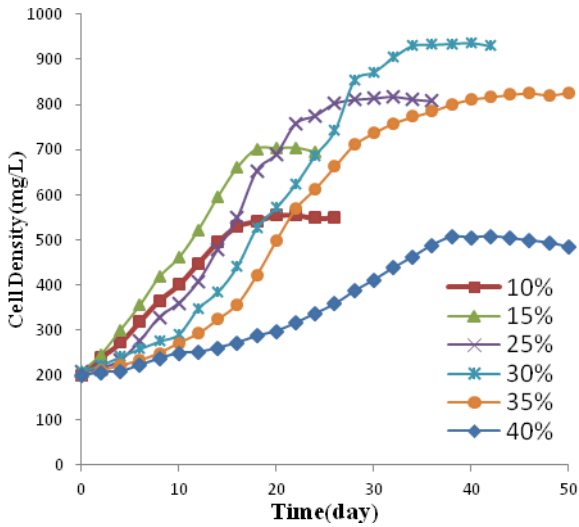
圖 11. 不同濃度 CO 2 連續曝氣下，小球藻的生長曲線
