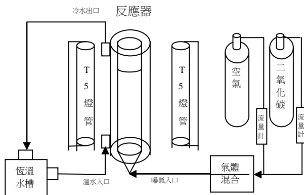
圖 2. 微藻培養設備
