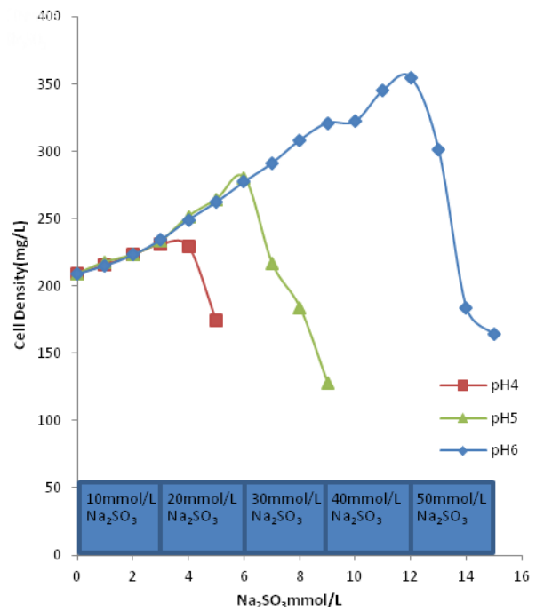
圖 12. 連續曝氣 CO 2 小球藻對 Na 2 SO 3 忍受力
