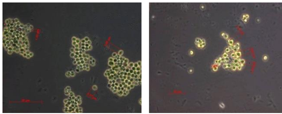
圖 1. 光學顯微鏡下的小球藻 (放大倍率 1000)
