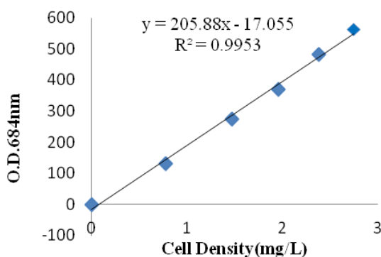
圖 3. 小球藻檢量線
