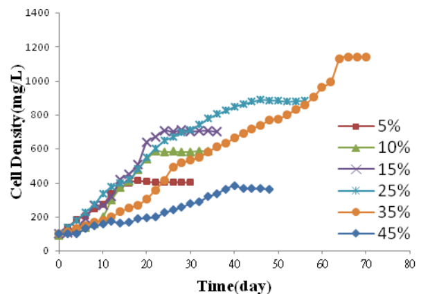
圖 4. 不同 CO 2 濃度下小球藻之生長曲線
