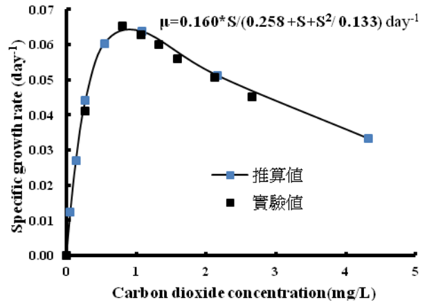
圖 6. 不同 CO 2 濃度培養下，小球藻之 Haldane 比生長速率曲線
