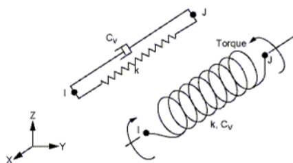
圖 3. Combin14 元素
