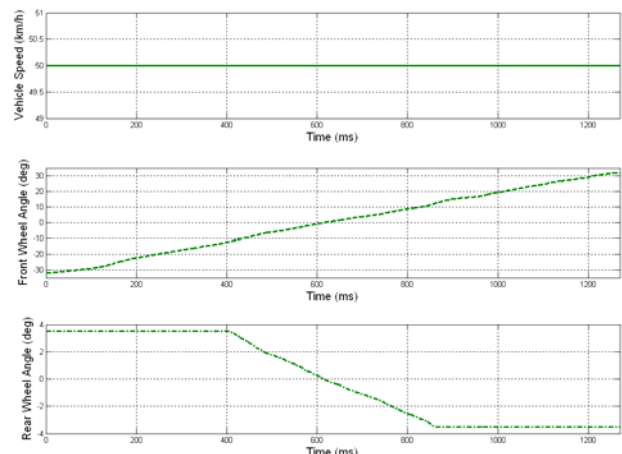
圖 21. 車速 50 km/h 時後輪逆相位轉向
