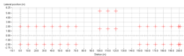
圖 9. 變換車道測試路線 [6]
