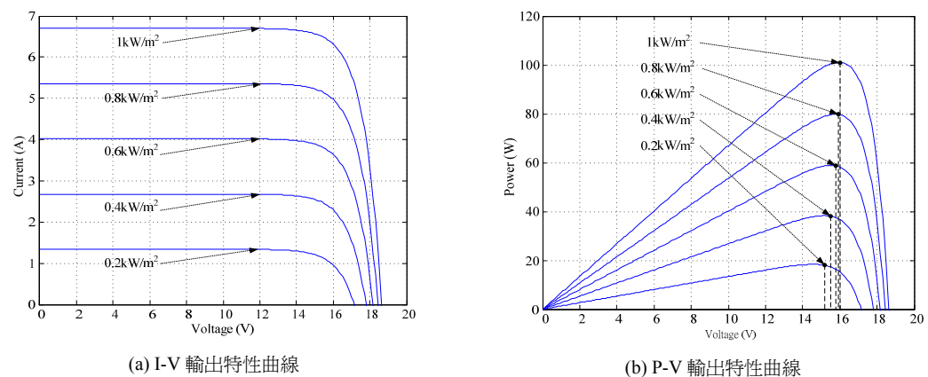
圖 10. V 型槽聚光型太陽光電模組在不同日照強度輸出特性曲線圖
