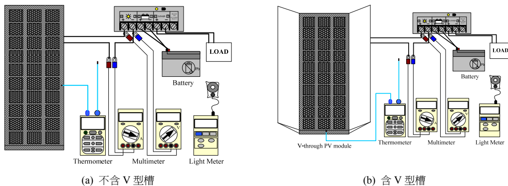
圖 12. 設備儀器配置圖
