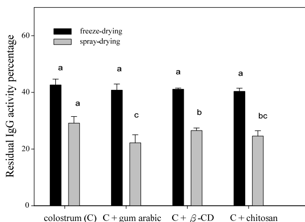
圖 1. 以不同乾燥法進行微膠囊化所得初乳之 IgG 殘存活性
