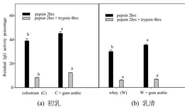
圖 9. 未微膠囊化及以阿拉伯膠微膠囊化之初乳與乳清經胃蛋白酶和胰蛋白酶水解後，再經 E. coli O55:B5 脂多醣作用後之 IgG 殘存活性
