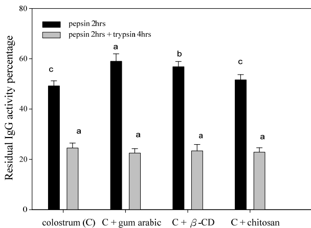
圖 6. 初乳及微膠囊化初乳以胃蛋白酶作用 2 小時及胰蛋白酶作用 4 小時後之 IgG 殘存活性
