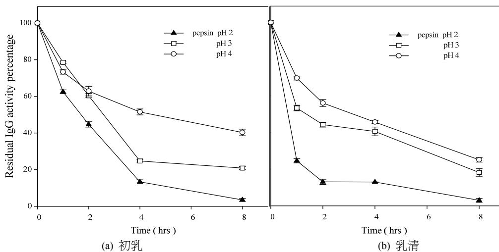
圖 5. 初乳和乳清於不同 pH 值下經胃蛋白酶作用 1、2、4、8 小時後之 IgG 殘存活性
