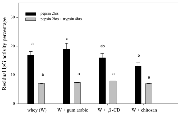
圖 7. 乳清及微膠囊化乳清以胃蛋白酶作用 2 小時及胰蛋白酶作用 4 小時後之 IgG 殘存活性
