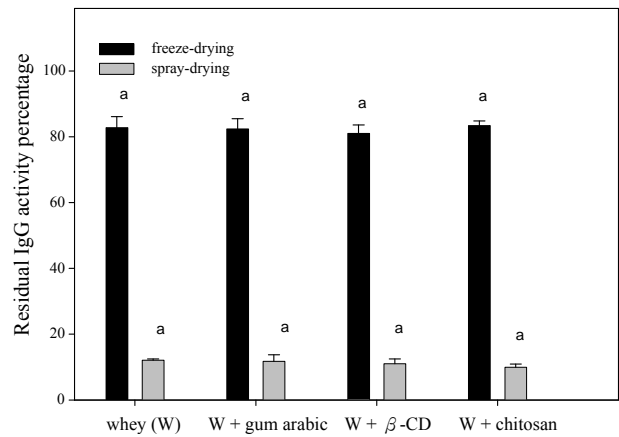
圖 2. 以不同乾燥法進行微膠囊化所得乳清之 IgG 殘存活性
