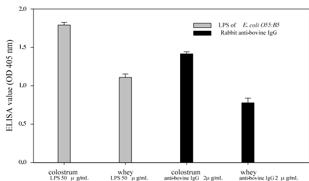
圖 8. 初乳與乳清經 E. coli O55:B5 脂多醣及兔子抗牛血清 IgG 反應後之 ELISA 值
