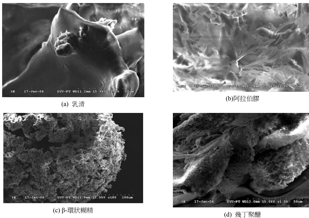
圖 4. 乳清、阿拉伯膠、 \beta -環狀糊精與幾丁聚醣膠囊化之乳清掃描式電子顯微照片
