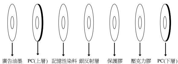
圖 1. DVD-R 光碟片之構造圖
