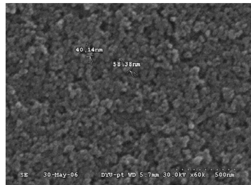
圖 5. TiO 2 工作電極孔洞特性
